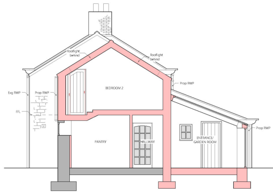
Section A-A, 1:50
